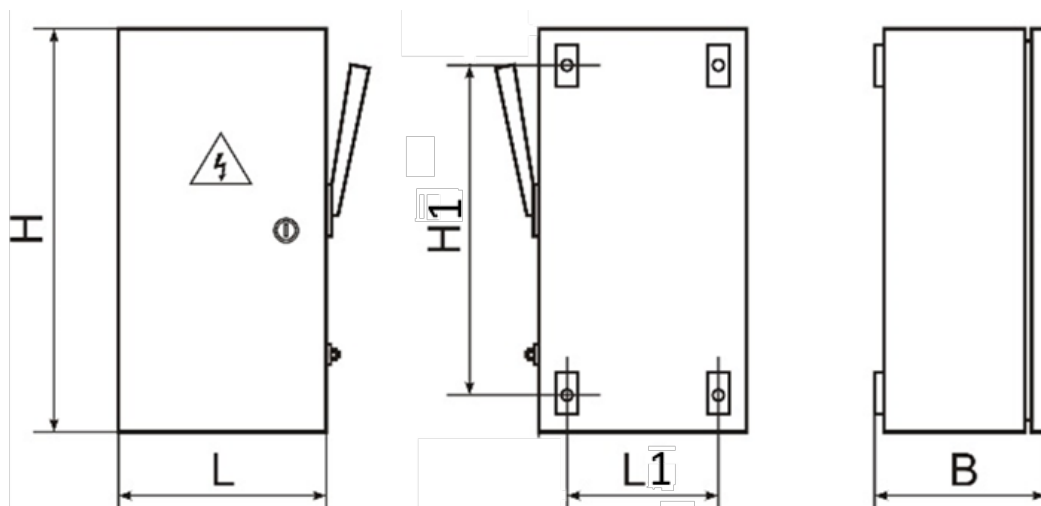
Рисунок 2. Габаритные и установочные размеры ящиков силовых ЯБПВУ-М.
