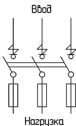
Принципиальная электрическая схема силовых ящиков серии ЯВЗ.
