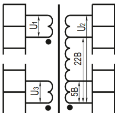
а) Трёхобмоточный трансформатор ОСМ1 с ответвлениями на вторичной обмотке
