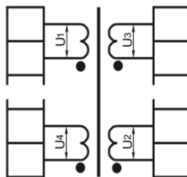
г) Четырёхобмоточный трансформатор ОСМ1
