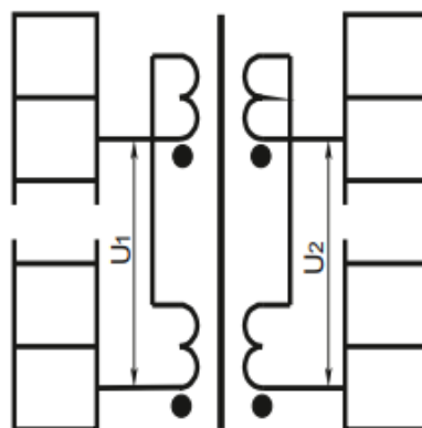
д) Двухобмоточный трансформатор ОСМ1
