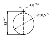
Рисунок 11. Размеры установочного отверстия в панели для установки выключателей кнопочных КЕ
