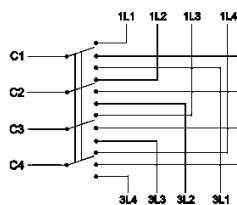
Пакетный переключатель ПП 4-полюсный на 3 направления
