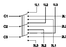
Пакетный переключатель ПП 3-полюсный на 3 направления
