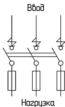
Принципиальная электрическая схема силовых ящиков серии ЯРВ.
