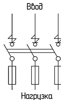
Рисунок 2. Схема электрическая принципиальная ЯРВ
