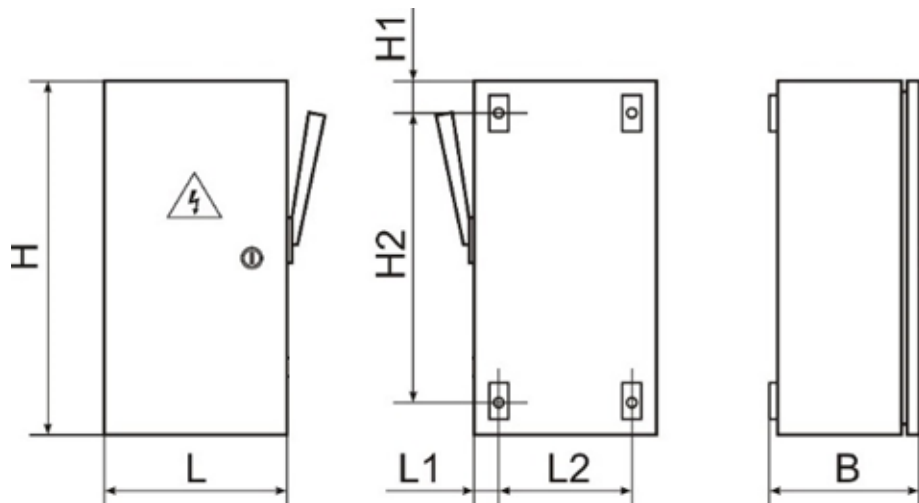
Рисунок 1. Общий вид и габаритные размеры ЯРВ
