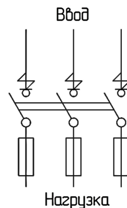
Рисунок 2. Схема электрическая принципиальная ЯВЗ
