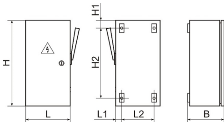
Рисунок 1. Общий вид и габаритные размеры ЯВЗ
