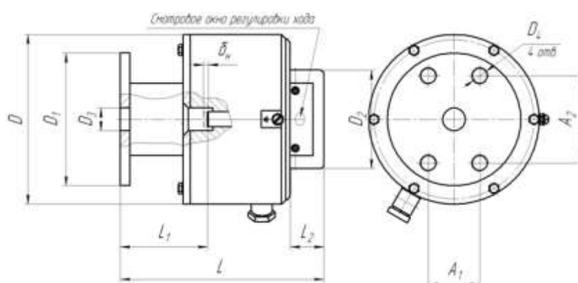
Рисунок 2. МП-301
