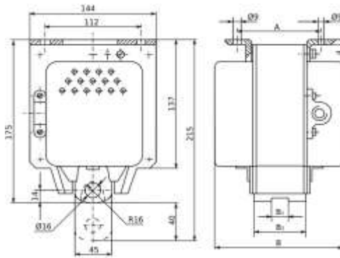
Рисунок 2. ЭД-10102, ЭД-11102
