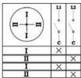
Рисунок 13. Пакетный переключатель 1-полюсный 4C
