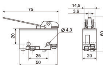
МП 2106М UXL3 исп.01.1А
