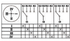
Рисунок 10. Пакетный переключатель 3-полюсный на 4 направления
