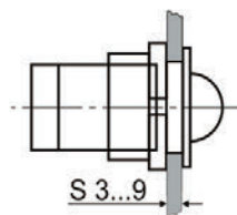
Крепление к панели
