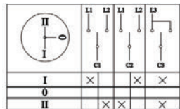
Рисунок 12. Пакетный переключатель 3-полюсный реверсный
