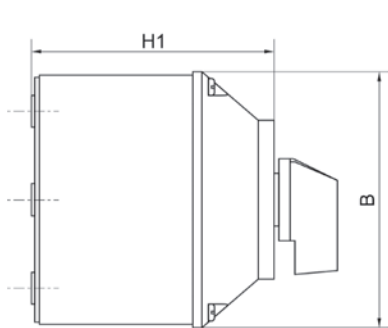
Рисунок 3. Габаритные размеры переключателя закрытого исполнения – РК.
