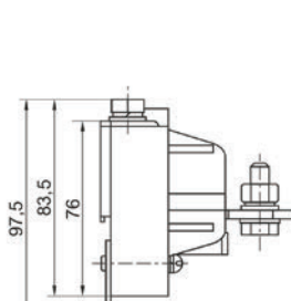
Реле для подключения к контактору
