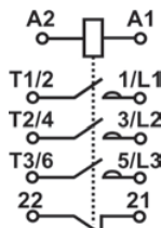
Рисунок 19. ПМЛ с доп.конт. 1p
