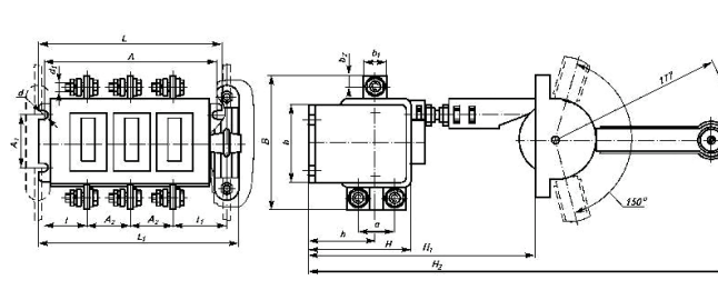
Рисунок 2в. BP32 с передней смещенной рукояткой, 2 направления
