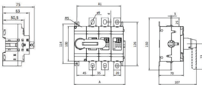
Рисунок 2. ВНК-160А3-20 УХЛ3, ВНК-250А3-20 УХЛ3
