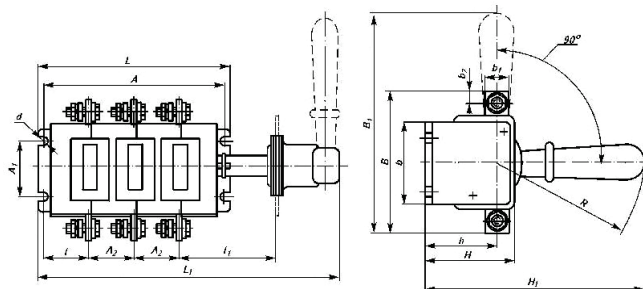
Рисунок 1б. BP32 с боковой смещенной рукояткой, 1 направление
