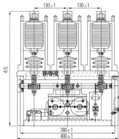
Рисунок 1. Габаритные размеры KBT-6
