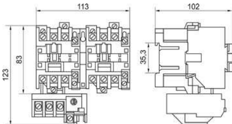
Пускатель реверсивный типа ПМ12-025
