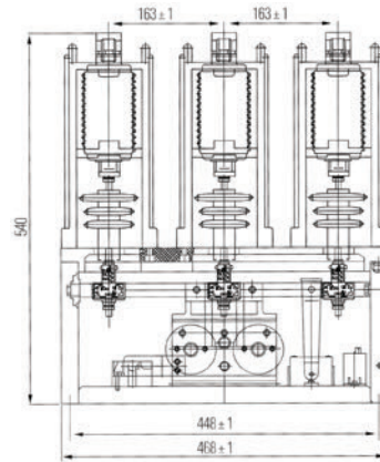
Рисунок 2. Габаритные размеры KBT-10
