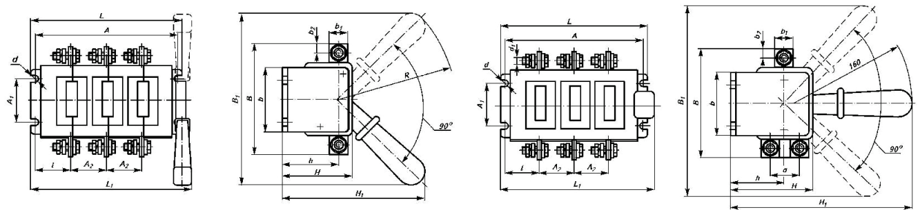
Рисунок 1а. BP32 с боковой рукояткой, 1 направление
