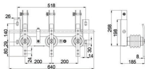
ЗР-10/400 УХЛ2; ЗР-10/630 УХЛ2; ЗР-10/1000 УХЛ2
