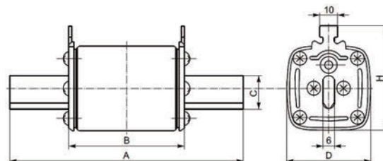
ППН-35, ППН-37, ППН-39
