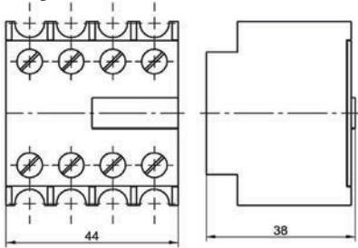
ПКЛ-04; ПКЛ-22; ПКЛ-31; ПКЛ-40
