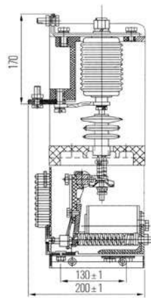
Рисунок 1. Габаритные размеры KBT-6
