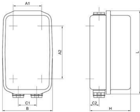
Рисунок 3. Пускатель серии ПМА, IP40
