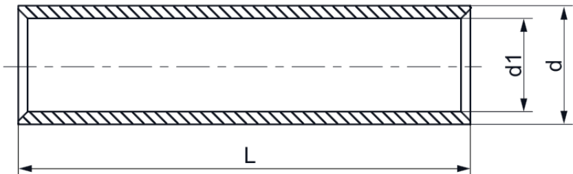
Рисунок 1. Общий вид и габаритные размеры.
