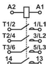
Рисунок 18. ПМЛ с доп.конт. 1z
