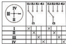
Рисунок 9. Пакетный переключатель 2-полюсный на 4 направления
