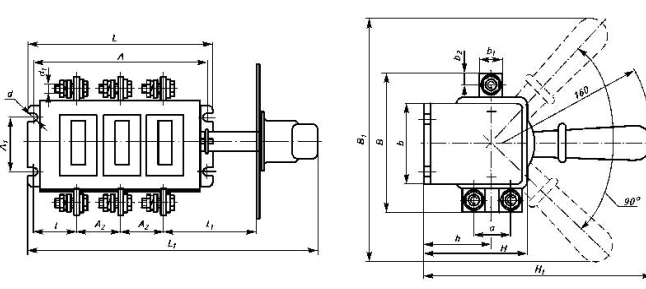
Рисунок 2б. BP32 с боковой смещенной рукояткой, 2 направления
