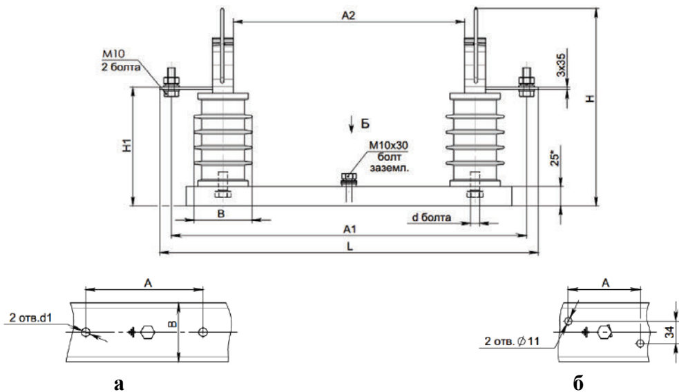
Рисунок 5. Габаритные, присоединительные и установочные размеры основания.
