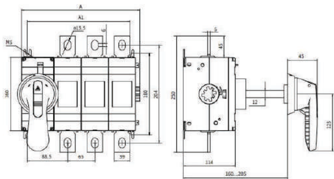
Рисунок 7. ВНК-630В3-20 УХЛЗ, ВНК-800В3-20 УХЛЗ
