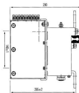
Рисунок 6. Габаритные размеры КВТ-1,14-1000/1250
