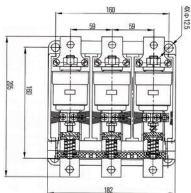
Рисунок 3. Габаритные размеры КВТ-1,14-250
