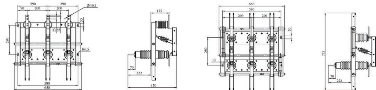
РВФЗ-10/630 II-II УЗ; РВФЗ-10/1000 II-II УЗ
