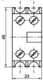
ПКЛ-02; ПКЛ-11; ПКЛ-20
