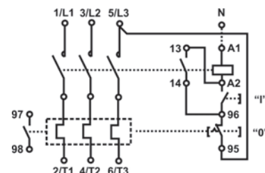
Рисунок 23. ПМЛ в оболочке с реле
