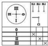
Рисунок 5. Пакетный переключатель 1-полюсный на 3 направления
