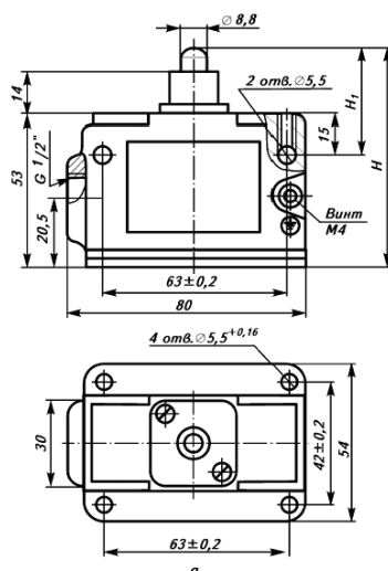
Рисунок 5. Общий вид, габаритные и установочные размеры микропереключателей МП1000 степень защиты IP54
