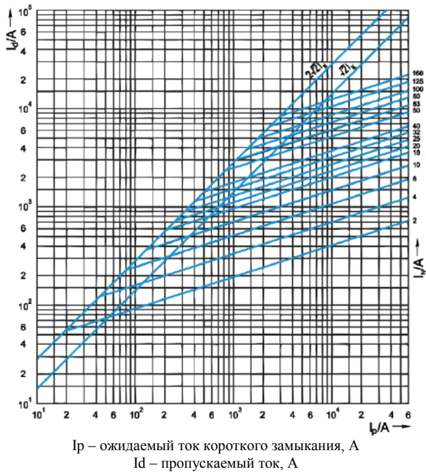
Рисунок 1. График тока отсечки для высоковольтных предохранителей серии ПКТ-VK
