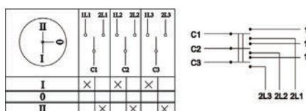
Рисунок 3. Пакетный переключатель 3-полюсный на 2 направления
