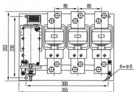
Рисунок 5. Габаритные размеры КВТ-1,14-630
