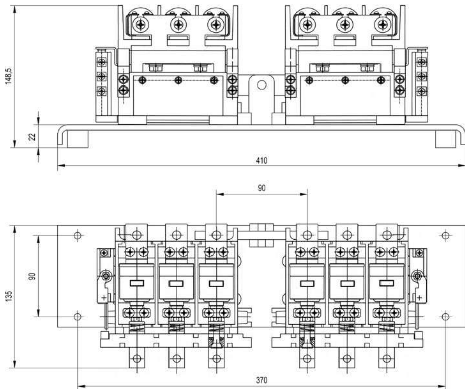
Рисунок 7. Габаритные размеры КВТ(Р)-1,14-80/125/160
