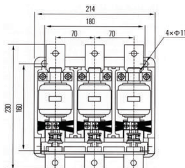
Рисунок 4. Габаритные размеры КВТ-1,14-400
