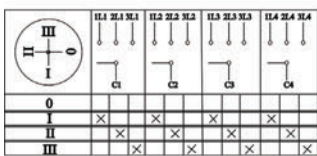
Рисунок 8. Пакетный переключатель 4-полюсный на 3 направления
