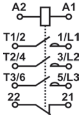
Рисунок 5. ПМЛ с доп.конт. 1p
