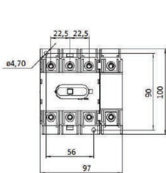
Рисунок 1. ВНК-63А3-20 УХЛ3, ВНК-100А3-20 УХЛ3, ВНК-125А3-20 УХЛ3
