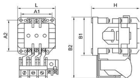
Рисунок 1. Пускатель серии ПМА-3000 нереверсивный с реле
