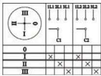
Рисунок 6. Пакетный переключатель 2-полюсный на 3 направления
