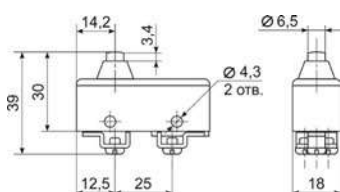
МП 2102Л UXL3 исп.03.1А
