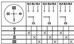
Рисунок 7. Пакетный переключатель 3-полюсный на 3 направления
