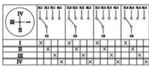
Рисунок 11. Пакетный переключатель 4-полюсный на 4 направления
