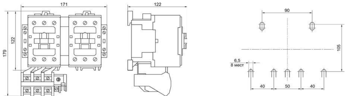
Пускатель реверсивный типа ПМ12-063
