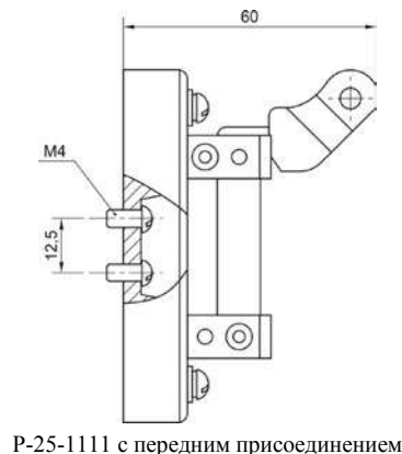
Р-25-1111 с передним присоединением
