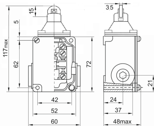
Рис.2. ВПК-2011-БУ2 - привод толкатель с роликом
