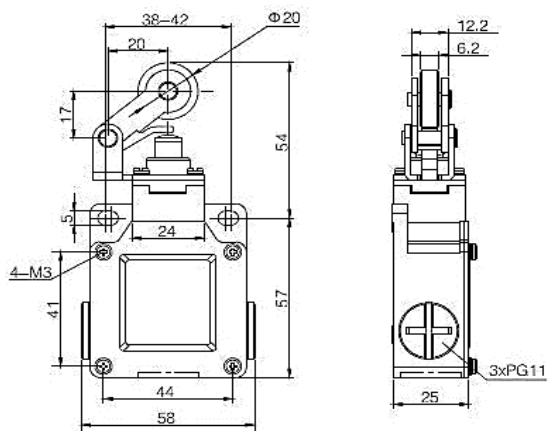
ВП 40-2121/23 (рычаг с роликом горизонтального срабатывания)
