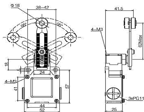
ВП 40-2143/45 (рычаг с роликом, регулируемый по длине)
