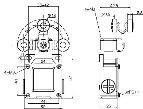
ВП 40-2116/18 (рычаг с роликом)
