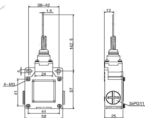
ВП 40-2106 (рычаг пружинный "кошачий ус")
