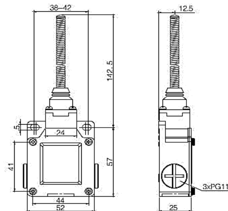
ВП 40-2108 (рычаг пружинный)
