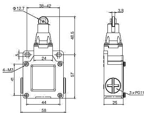
ВП 40-2102 (толкатель с роликом)
