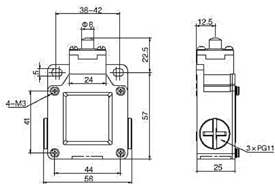
ВП 40-2110 (толкатель)
