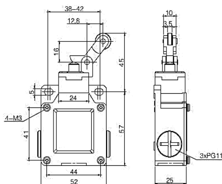
ВП 40-2127 (рычаг с роликом вертикального срабатывания)
