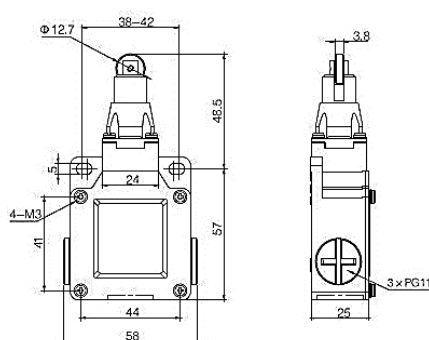
ВП 40-2102 (толкатель с роликом)
