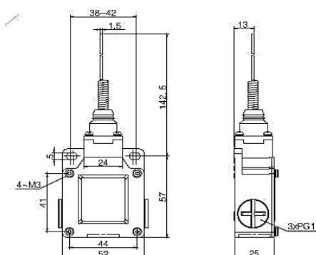
ВП 40-2106 (рычаг пружинный \"кошачий ус\")
