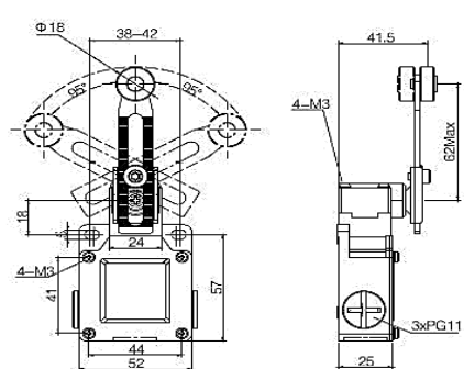
ВП 40-2143/45 (рычаг с роликом, регулируемый по длине)
