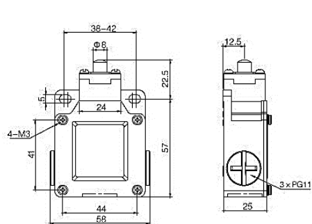
ВП 40-2110 (толкатель)
