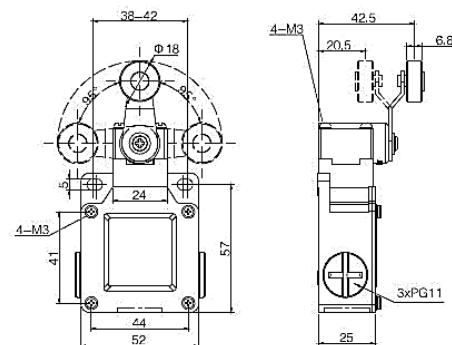
ВП 40-2116/18 (рычаг с роликом)
