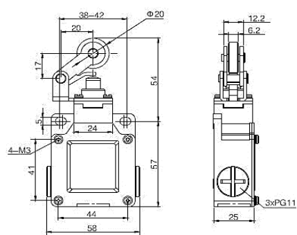
ВП 40-2121/23 (рычаг с роликом горизонтального срабатывания)
