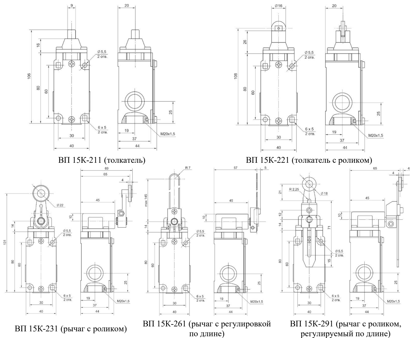
Рисунок 2. Габаритные и установочные размеры путевых выключателей.
