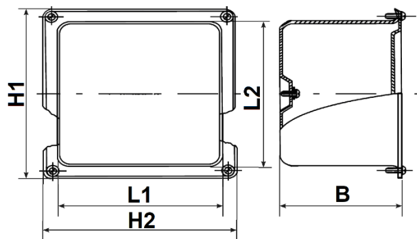
Рисунок 1. Габаритно-установочные размеры
