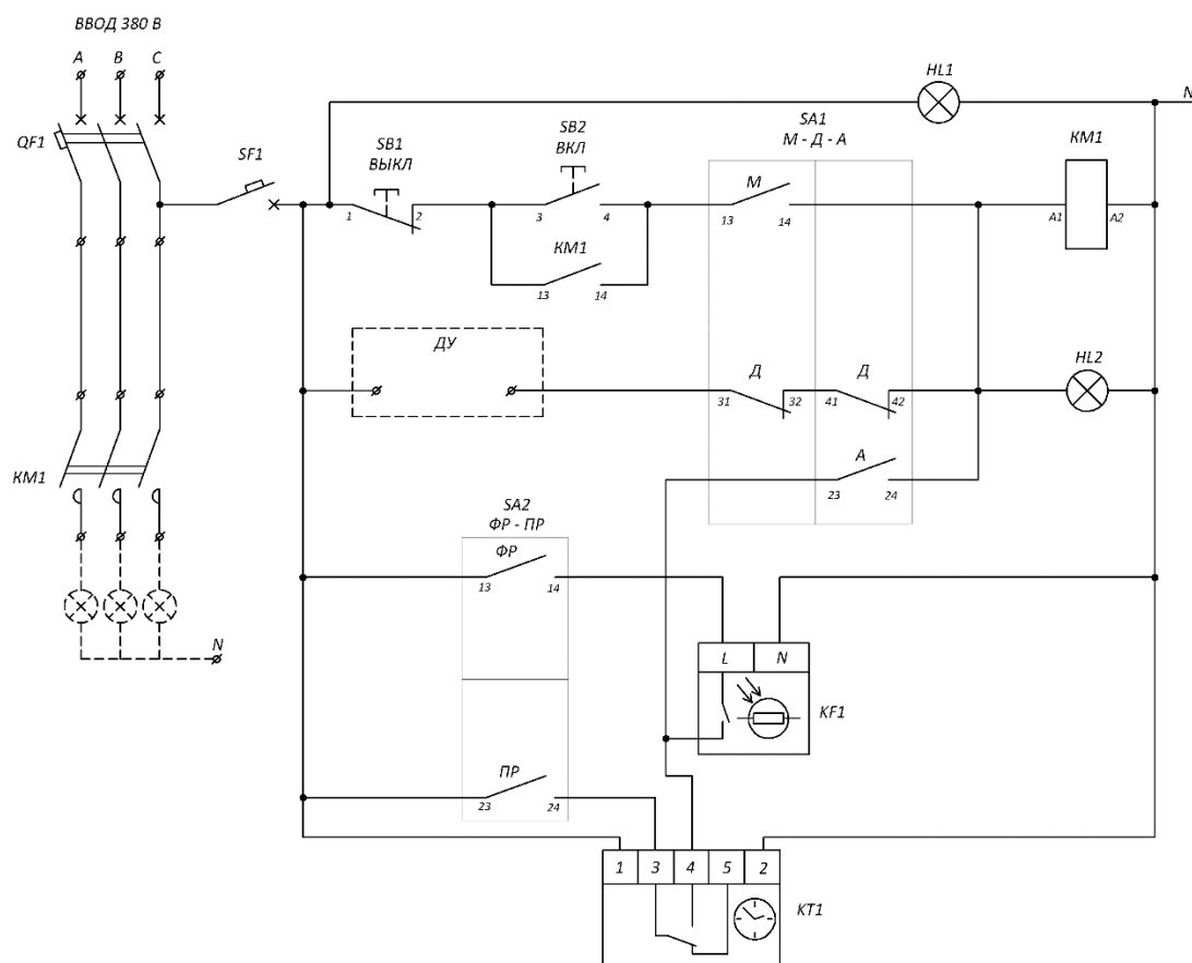
Рисунок 1. Принципиальная электрическая схема ЯУО-9601 (с программатором и фотореле)
