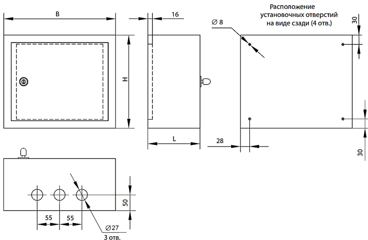
Рисунок 4. Габаритные и установочные размеры ящиков управления освещением
