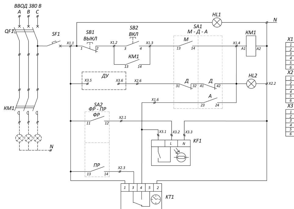
Рисунок 2. Принципиальная электрическая схема ЯУО-9601
