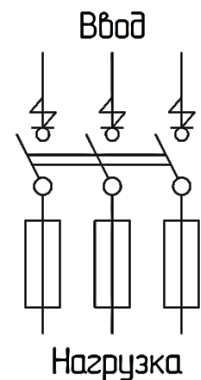
Рисунок 2. Схема электрическая принципиальная ЯРП
