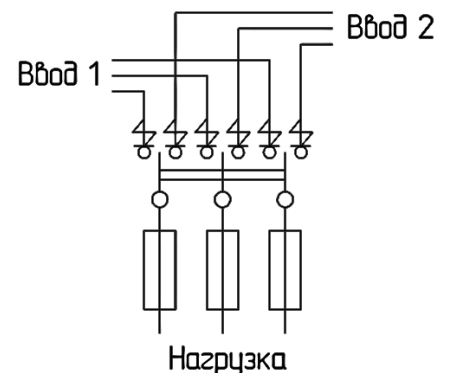
Рисунок 4. Схема электрическая принципиальная ЯРПП
