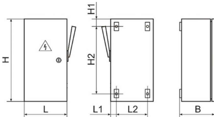
Рисунок 1. Общий вид и габаритные размеры ЯРП
