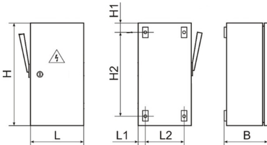
Рисунок 3. Общий вид и габаритные размеры ЯРПП
