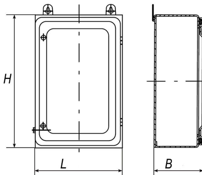
Рисунок 1. Габаритно-установочные размеры ящиков протяжных серии K650
