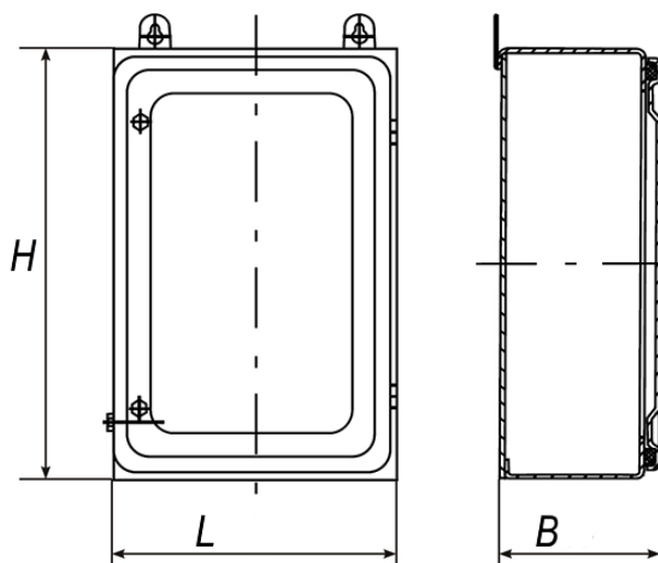
Габаритно-установочные размеры ящиков протяжных серии K650
