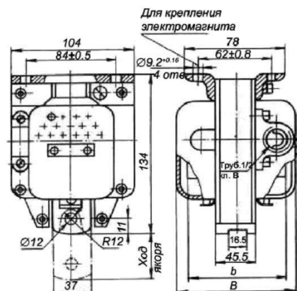
Рисунок 6. Габаритные размеры электромагнита МИС-6100
