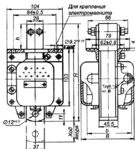
Рисунок 7. Габаритные размеры электромагнита МИС-6200
