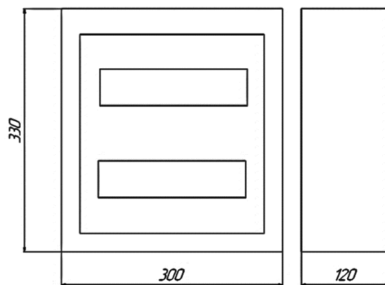
Рисунок 2. Габаритные и установочные размеры щитков осветительных ОЦВ-12
