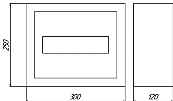
Рисунок 1. Габаритные и установочные размеры щитков осветительных ОЦВ-6
